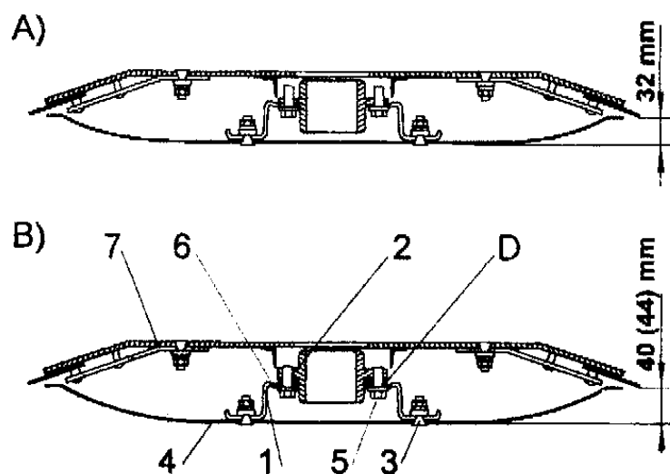
Рис. 13. Установка высоты скашивания а) низкая 32 мм (без дистанционного кольца D), б) средняя 40 мм (с дистанционным кольцом D)
